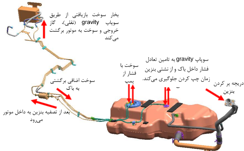
شمای کلی سیستم کنترل آلایندگی بخار سوخت
